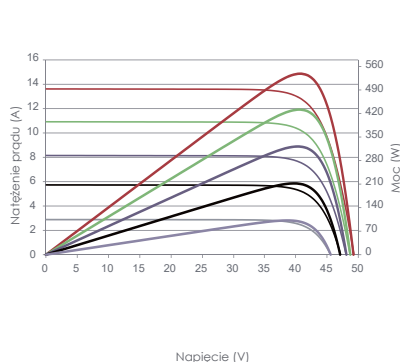
Krzywe prądowo-napięciowe i mocowo-napięciowe (540W)
